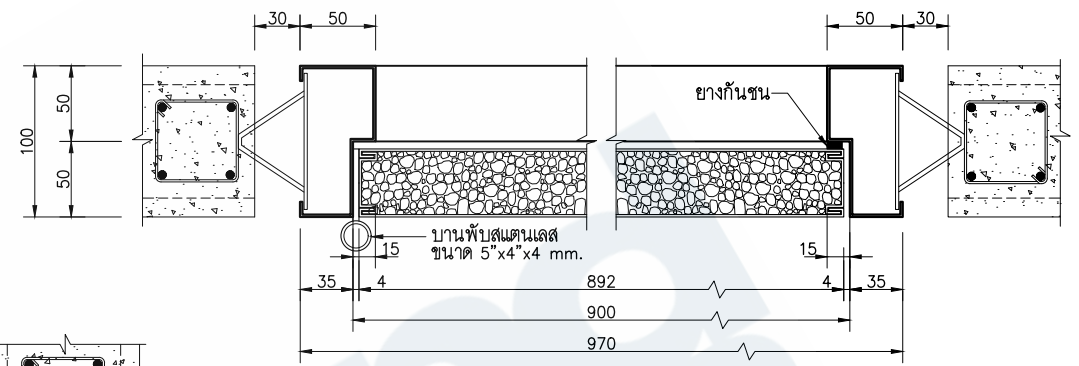
รูปตัด SCALE 1:5 (A4)
