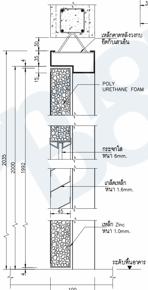
รูปตัด SCALE 1:5 (A4)
