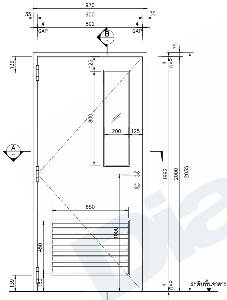
รูปด้านหน้า SCALE 1:20 (A4)
