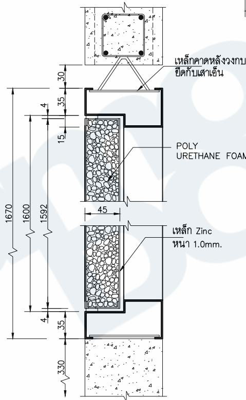
รูปตัด SCALE 1:5 (A4)
