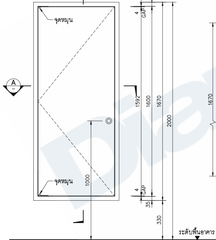
รูปด้านหน้า SCALE 1:20 (A4)
